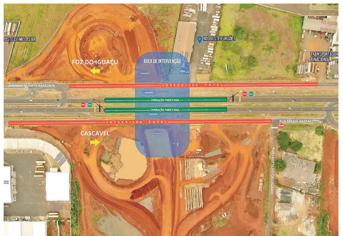
Serão lançadas por guindaste 12 vigas longarinas sobre os pilares do viaduto DER-PR
